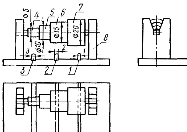
1 - 7 - стержни; 8 - стойка
